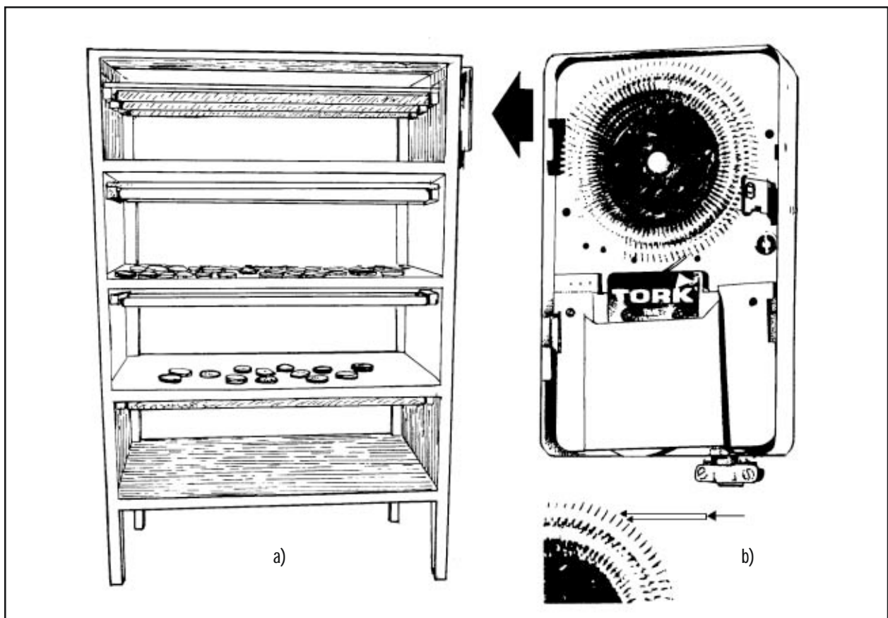
Figura 3 a. Cámara de crecimiento de construcción artesanal. b. Reloj control para regular la iluminación.
