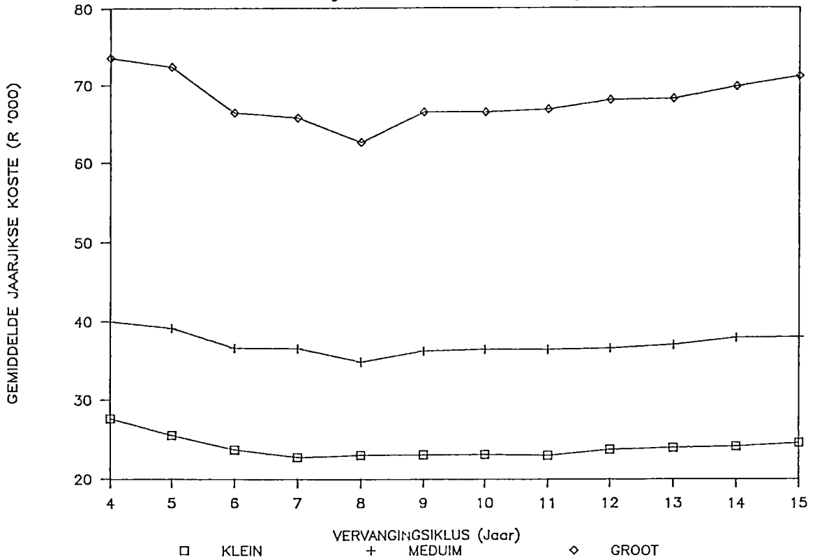
Figuur 4 : Die effek van trekkergrootte en vervangingsiklus op gemiddelde jaarlikse koste
